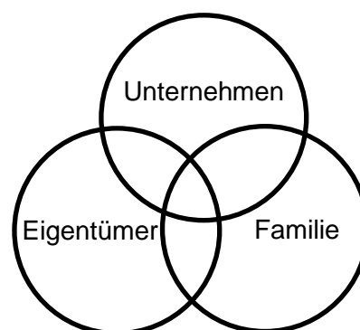
Abbildung 3: Drei-Kreise-Modell.
